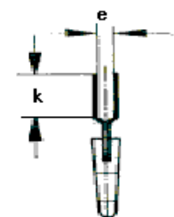
Juotoshaarukka:
